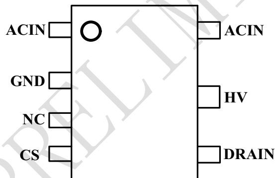
图 2 管脚封装图
